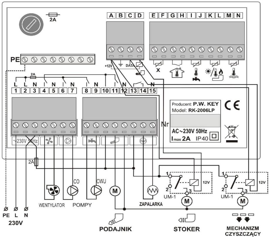
Rysunek 2. Schemat podłączenia regulatora RK-2006LP.
